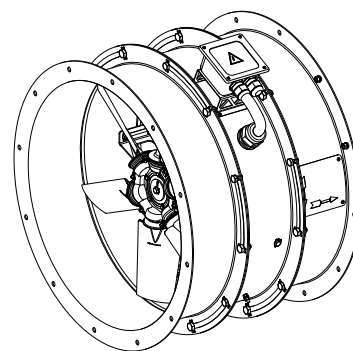
Рисунок 1.2 – Корпус 10.20
